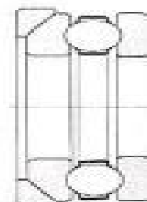
11b. Kogeltaetsl. met bolle huisring en insceiding
